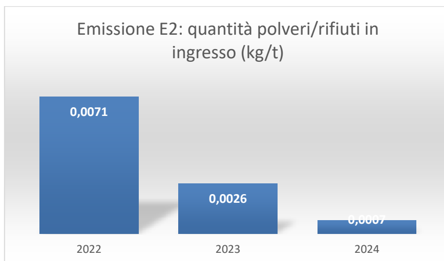
Figura 14 – E2: quantità di polveri rispetto alla quantità di rifiuti gestiti (fonte: rapporti di prova MP Labs n. 2609/4-5-6 del 21.06.24)
