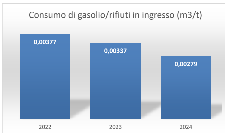
Figura 19 – Consumi di gasolio rispetto alla quantità di rifiuti gestiti (fonte: fatture di acquisto gasolio registrate dall'amministrazione)
