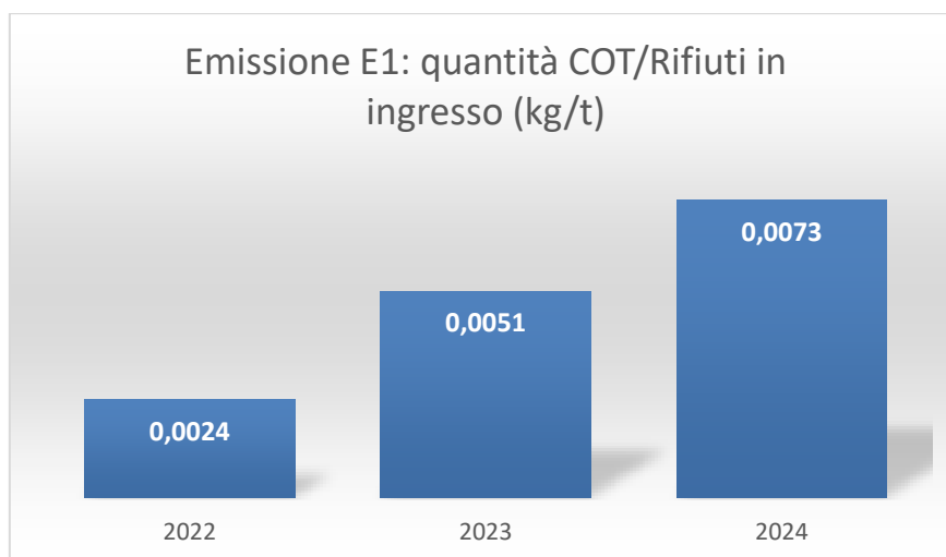
Figura 13 – E1: quantità di COT rispetto alla quantità di rifiuti gestiti (fonte: rapporti di prova MP Labs n. 2609/1-2-3 del 21.06.24)
